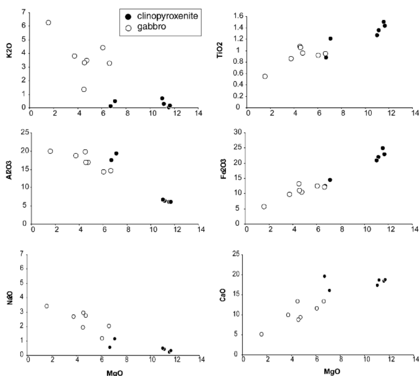
شکل ۲ نمودارهای تغییرات اکسید عناصر اصلی نسبت اکسید منیزیم در واحدهای مافیک و اولترامافیک مجموعه‌ی آذرین هشت سر. اکسیدهای \text{CaO} , \text{Fe}_2\text{O}_3 , \text{TiO}_2 با منیزیم را بطنی مستقیم و \text{K}_2\text{O} , \text{Al}_2\text{O}_3 , \text{Na}_2\text{O} با آن رابطه عکس دارند.
