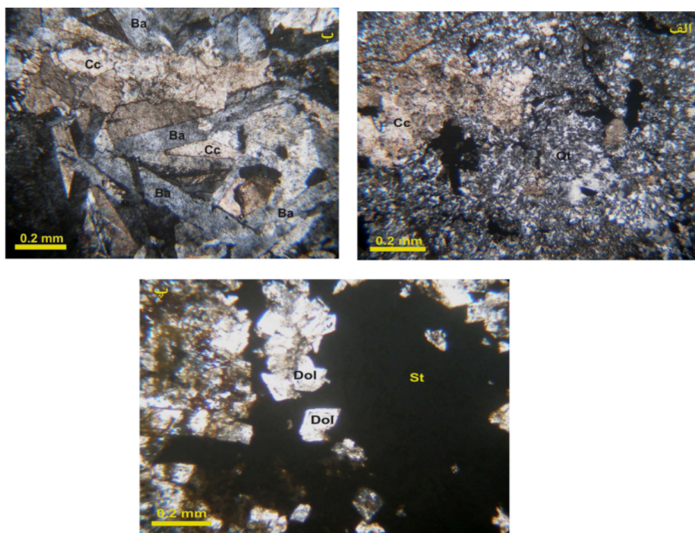
شکل ۸ تصاویر میکروسکوپ از دگرسانی سنگ میزبان الف) سیلیسی شدن سنگ آهک (نمونه‌ی Si-19 نور XPL)، ب) تیغه‌های درشت باریت همراه با کلسیت درشت بلور (نمونه‌ی Si-30 نور XPL)، پ) بلورهای لوزی شکل دولومیت که پیش از استیبنیت تشکیل شده است (نمونه‌ی Si-35 نور XPL). Qt = کوارتز، Cc = کلسیت، Ba = باریت، Dol = دولومیت، St = استیبنیت.
