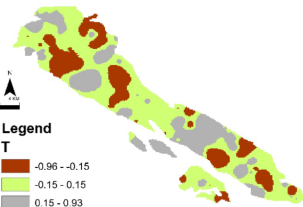
شکل ۷ نقشه‌ی پربندی مقادیر T برای توده‌ی گرانیتوئیدی بروجرد.
