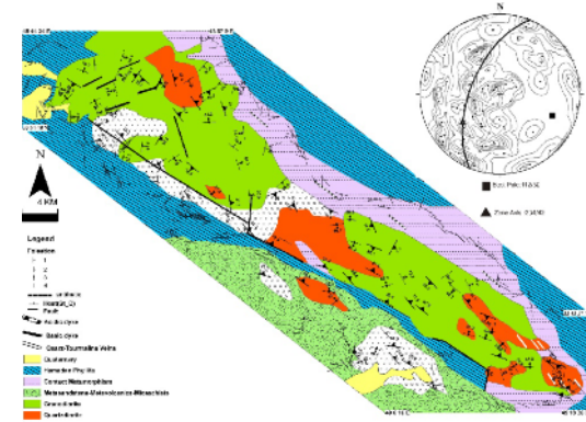
شکل ۱۱ محل برگوارگی‌های مغناطیسی روی نقشه‌ی توده گرانیتوئیدی بروجرد. که هر کدام از پهنه‌های چهارگانه به ترتیب با شماره ۱ تا ۴ و با نماد متفاوت مشخص شده‌است.
