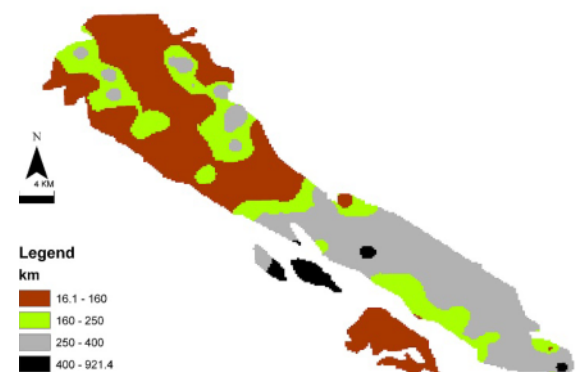
شکل ۶ نقشه‌ی پربندی مقادیر Km برای همبافت گرانیتوئیدی بروجرد.
