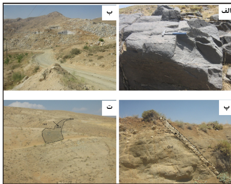
شکل ۲ الف: نمایی از گرانودیوریت های منطقه‌ی مورد بررسی ب: نمایی از مونوزودیوریت های گوشه که به دلیل عدم هوازدگی و تازه گی و خوش رنگ بودن به صورت سنگ ساختمانی استخراج می‌شود. پ: نمایی از یک رگه‌ی پگماتیتی که در درون واحد گرانودیوریتی تزریق شده است. ت: نمایی از یک دایک بازی، Grd گرانودیوریت، Dy.M دایک بازی.
