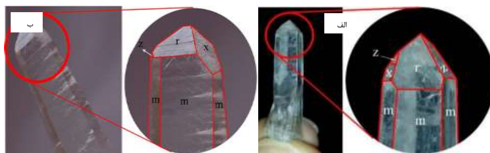
شکل ۵ (الف) شکل راست گرد بلور کوارتز قهرود، (ب) چپ گرد در بلور کوارتز قهرود.
