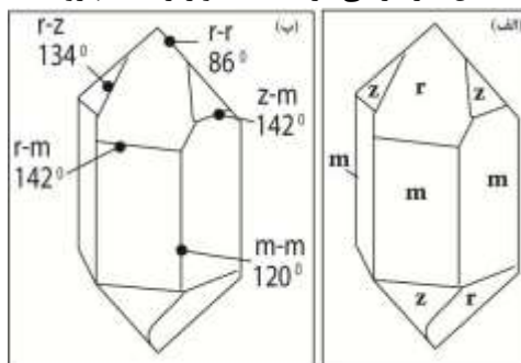
شکل ۳ (الف) بلور کوارتز معمولی با سطوح مشخص r , z , m , (ب) زاویه‌ی بین سطح در بلور کوارتز معمولی [۸].
