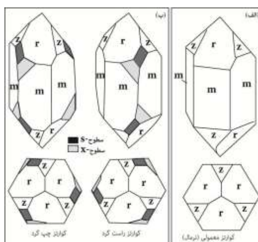
شکل ۴ (الف) موقعیت سطوح r و z در کوارتز معمولی، (ب) تعیین راست گرد و چپ گرد بودن کوارتز با استفاده از سطوح s , x [۸].
