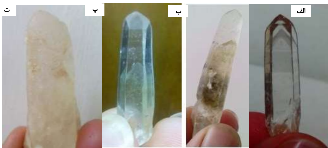
شکل ۱۳ (الف-پ) شکل فانوم در بلورهای کوارتز قهرود، (ت) شکل نیمه استلاگمیتی در بلورهای کوارتز قهرود.
