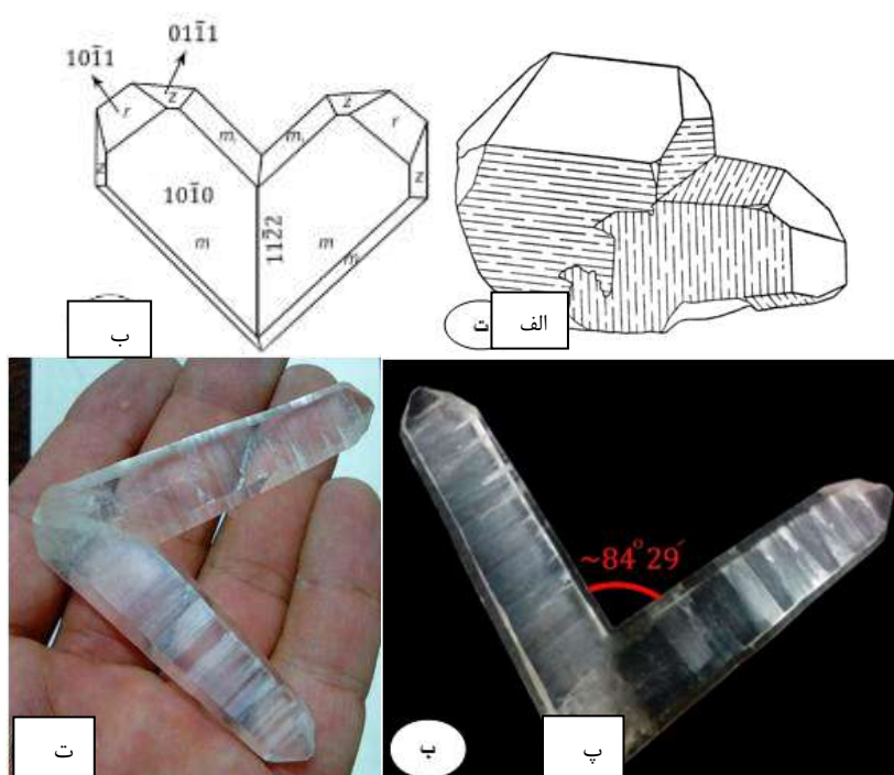
شکل ۱۶ دوقلویی با قاعده‌ی ژاپنی در بلورهای کوارتز. (الف) سطح مشترک جدا کننده دو بلور کوارتز با قاعده ژاپن بصورت خطی و صاف است [۱۱]، (ب) مرز غیر خطی در دو کوارتز با قاعده‌ی ژاپن [۱۱]، (پ) کوارتز شناسایی شده با ماکل قاعده‌ی ژاپن در منطقه قهرود (اندازه هر بلور کوارتز در حدود ۷ سانتی متر است)، (ت) دوقلویی در کوارتز قهرود با قاعده ژاپن. زاویه‌ی اندازه گیری شده بین دو سطح متصل به هم تقریباً برابر با ۸۴ درجه و ۲۹ دقیقه است.
