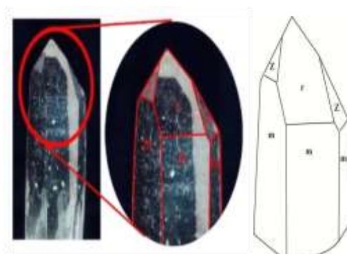
شکل ۵ (الف) شکل راست گرد بلور کوارتز قهرود، (ب) چپ گرد در بلور کوارتز قهرود.
