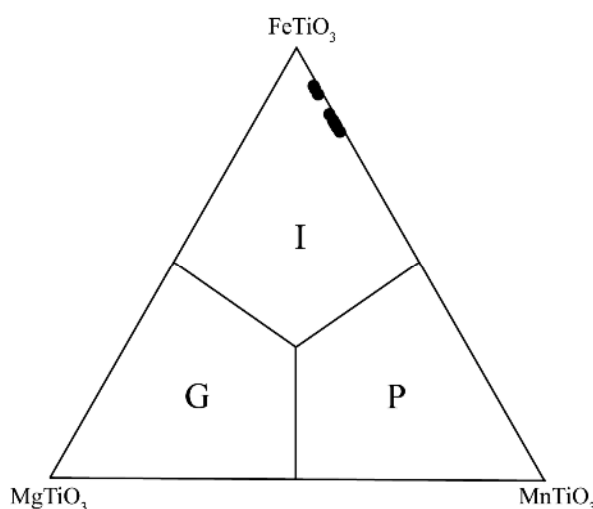
شکل ۶ ترکیب شیمیایی ایلمنیت موجود در گرانیتهای شیرکوه در نمودار \text{FeTiO}_3 ، \text{MnTiO}_3 و \text{MgTiO}_3 . قلمروهای پیروفانیت (P)، ایلمنیت (I) و ژیکلیت (G) نیز نشان داده شده‌اند [۲۳].
