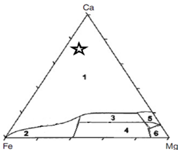
شکل ۱۲ تشخیص خاستگاه تورمالین براساس نمودار مثلثی پرستون و همکاران (۲۰۰۲) [۲۸]، ستاره موقعیت تورمالین‌های ناحیه‌ی مورد بررسی را نشان می‌دهد. (ناحیه‌ی ۱، گرانیتوئیدها، پگماتیت‌ها و اپلیت‌های غنی از Li. ناحیه‌ی ۲، گرانیتوئیدها، پگماتیت‌ها و اپلیت‌های فقیر از Li. ناحیه-۳، متاسامیت، متاپلیت‌ها و کلسی سیلیکات‌های غنی از Ca. ناحیه‌ی ۴، متاسامیت، متاپلیت‌ها و سنگ‌های تورمالین کوارتزی فقیر از Ca. ناحیه‌ی ۵، متاکربنات‌ها و ناحیه‌ی ۶، متاپیروکسینیت‌ها).
