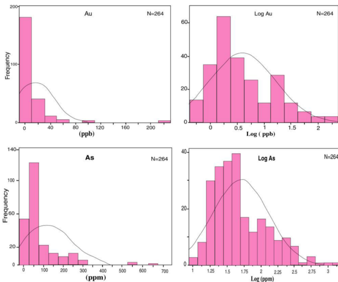
شکل ۶ نمودار ستونی داده‌های خام و لگاریتمی عناصر انتخابی Au, As در نمونه‌های خاک تاریک‌دانه.
