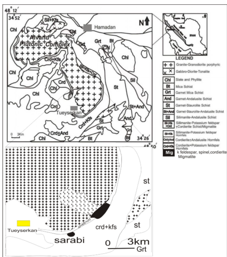
شکل ۱ موقعیت زمین‌شناسی منطقه‌ی مورد بررسی: موقعیت زون سندج- سیرجان و موقعیت منطقه‌ی مورد نظر را نشان می‌دهد اقتباس از [۲۳]. بخش پایین تصویر بخش‌هایی را که به وسیله ی گابرو دستخوش ذوب بخشی شده است را نشان می‌دهد.
