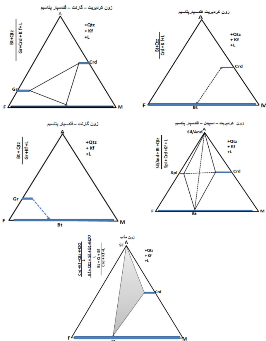
شکل ۴ روابط فازي و واکنش‌های دگرگونی در سنگ‌های رسی و نیمه رسی دگرگون منطقه سرابی.
