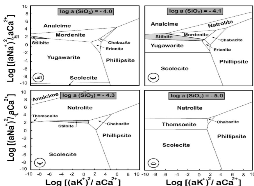
شکل ۱۲ نمودار تغییرات گستره‌ی پایداری ژئولیت‌ها با تغییر فعالیت سیلیس محلول (الف تا ت) [۱۹].
