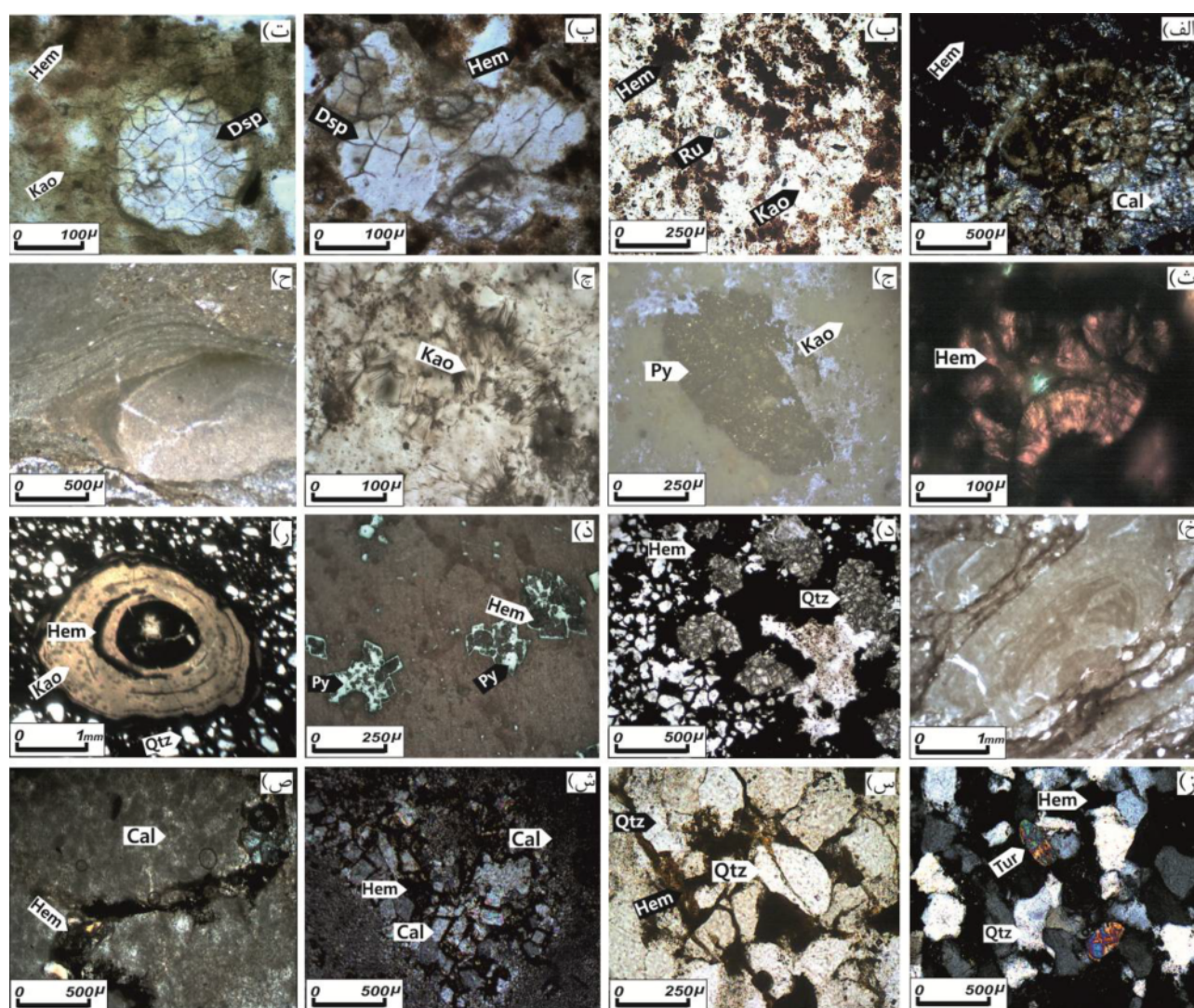
شکل ۶ تصاویر میکروسکوپی از واحدهای مختلف بوکسیتی در منطقه‌ی مورد بررسی. الف) آثار فسیلی گاستروپود در واحد بوکسیت بالایی، ب) ذرات آواری روتیل و آناتاز در واحد کائولینیت بالایی، پ) بافت برشی دروغین محدود به کانی‌های بوهمیت و دیاسپور، ت) بافت برشی دروغین در کانی‌ها و زمینه سنگ، ث) هماتیت ثانویه با بافت شعاعی در اطراف کانی‌های هماتیت، ج) گرهک‌های پیریتی در واحد کائولینیت پایینی، چ) کائولینیت‌های واحد بوکسیت پایینی، ح) بافت کلوفورمی-جریانی، د) بافت اسفنجی هماتیت و پرشدگی حفره‌ها به وسیله ی کوارتز ثانویه، ذ) بافت جعبه‌ای ناشی از دگرسانی پیریت و تبدیل آن به هماتیت، ر) بافت پیروئیدی، ز) بافت آرنایتی ناشی از ذرات تخریبی کوارتز و تورمالین که از شواهد نابرجاز بودن نهشته بوکسیتی است، س) پرشدگی شکستگی‌های کوارتز به وسیله ی هماتیت، ش، ص) پرشدگی شکستگی‌های موجود در سنگ آهک روته به وسیله ی کلسیت و اکسیدهای آهن ثانویه. تصاویر الف، ز، ش، ص، در نور عبوری قطبیده، تصاویر ج، ذ، در نور بازتابی عادی و تصاویر دیگر در نور عبوری عادی گرفته شده‌اند.
