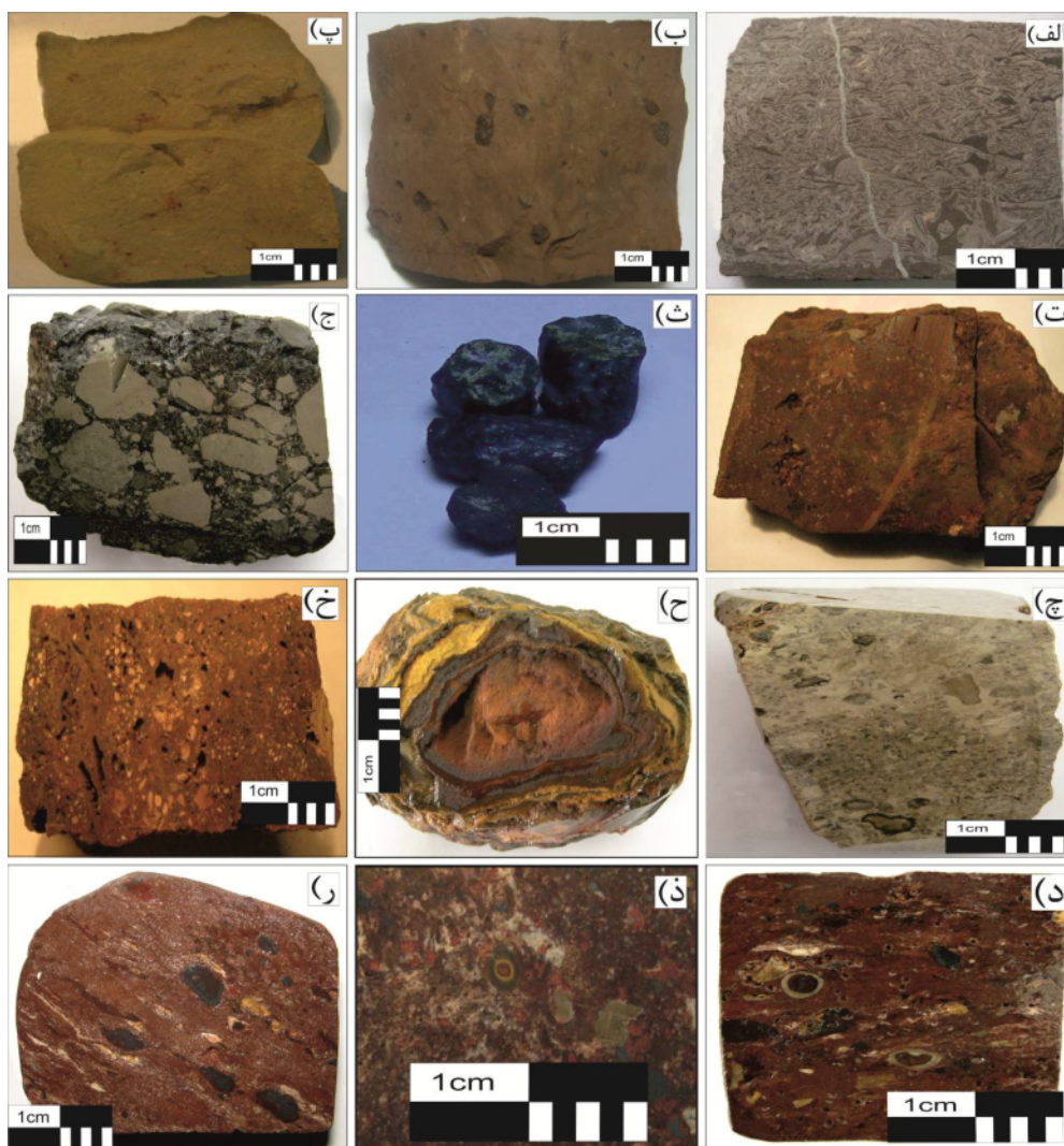
شکل ۵ تصاویر ماکروسکوپی واحدهای مختلف بوکسیتی در منطقه‌ی مورد بررسی، (الف) بافت ورمیکولار و حاوی فسیل گاستروپود در بالاترین بخش از واحد بوکسیت بالایی، (ب) بافت گرهکی در بوکسیت سرخ توده‌ای، (پ) بافت ریز دانه در واحد کائولینیت بالایی، (ت) نمونه‌ای از واحد بوکسیت سخت حاوی بوهمیت و دیاسپور، (ث) گرهک‌های استوانه‌ای شکل پیریتی در واحد کائولینیت پایینی که پس از جداسازی به روش XRD شناسایی شدند، (ج) بافت کاتاکلاستیک، (چ) نمونه‌ای از بوکسیت سفید سخت حاوی بوهمیت و دیاسپور در واحد کائولینیت پایینی، (ح) بافت گرهکی، (خ) بافت پرکننده فضاهای خالی، (د) بافت گرهکی و پیزوئیدی، (ذ) بافت پیزوئیدی، (ر) بافت گرهکی - جریانی.
