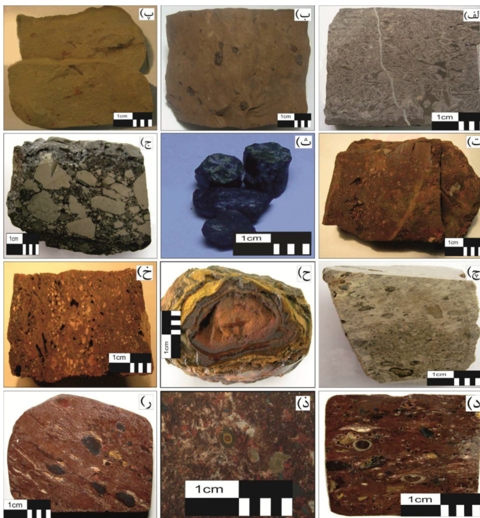
شکل ۵ تصاویر میکروسکوپی واحدهای مختلف بوکسیتی در منطقه‌ی مورد بررسی، الف) بافت ورمیکولار و حاوی فسیل گاستروپود در بالاترین بخش از واحد بوکسیت بالایی، ب) بافت گرهکی در بوکسیت سرخ توده‌ای، پ) بافت ریز دانه در واحد کائولینیت بالایی، ت) نمونه‌ای از واحد بوکسیت سخت حاوی بوهمیت و دیاسپور، ث) گرهک‌های استوانه‌ای شکل پیریتی در واحد کائولینیت پایینی که پس از جداسازی به روش XRD شناسایی شدند، ج) بافت کاتاکلاستیک، چ) نمونه‌ای از بوکسیت سفید سخت حاوی بوهمیت و دیاسپور در واحد کائولینیت پایینی، ح) بافت گرهکی، خ) بافت پرکننده فضاهای خالی، د) بافت گرهکی و پیزوئیدی، ذ) بافت پیزوئیدی، ر) بافت گرهکی - جریانی.
