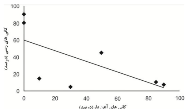
شکل ۹ مقادیر نیمه کمی کانی های آهن دار نسبت به کانی های رسی در نیمرخ شماره ۲.
