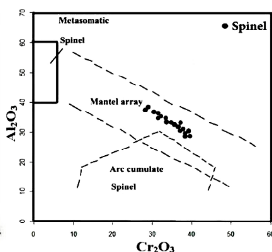
شکل ۷ الف: نمودار Al_2O_3 نسبت به Cr_2O_3 در اسپینل که خاستگاه گوشته ای اسپینل ها را نشان می دهد. [۲۳، ۲۲، ۲۱]. ب- Cr^{\#} اسپینل نسبت به Mg^{\#} الیوین های همزیست در پریدوتیت که نشان دهنده ترکیب OSMAs و abyssal است. [۲۴].
