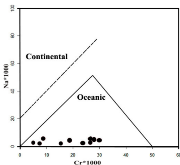
شکل ۹ مقدار اتمي Na کليوپيروکسن نسبت به Cr آن در پريدوتيت هاي گوشته‌اي منطقه [۲۶]، پريدوتيت‌هاي افيليت منطقه در گستره‌ي افيانوسي قرار مي گيرند.
