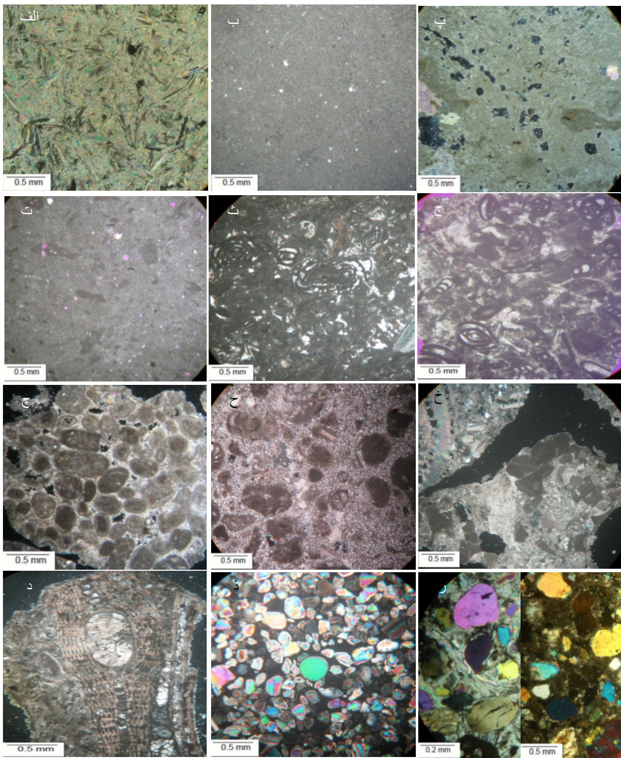
شکل ۳ الف) زیررخساره‌ی انیدریت، ب) زیررخساره‌ی مادستون کوارتز دار، پ) زیررخساره‌ی دولومادستون با بافت فنسترال، ت) زیررخساره‌ی مادستون بایوکلاست دار، ث) زیررخساره‌ی بورلیس-میلیولید بایوکلاست دار، ج) زیررخساره‌ی وکستون-پکستون بایوکلاست دار، خ) زیررخساره‌ی وکستون-پکستون حاوی فرامینیفرهای بنتیک، د) زیررخساره‌ی وکستون-پکستون لپیدوسیکیلینا، نومولیت، بیوکلاست دار، ذ) زیررخساره‌ی کوارتز آرنایت بدون سیمان، ر) زیررخساره‌ی کوارتز آرنایت با سیمان سولفاتی و سیمان دولومیتی.
