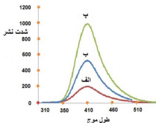
شکل ۱۶ طیف فلوئورسانس وابسته به متاسیلیکات سنتز لیتیم با نسبت \text{Li}:\text{Si} ۱:۲ از نیترات لیتیم و اسید سیلیسیک در طول زمان‌های (الف) ۴۸ ساعت، (ب) ۷۲ ساعت، (پ) ۹۶ ساعت.
