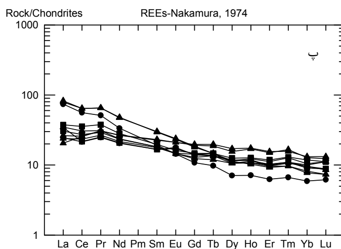
شکل ۷ پ- نمودار جریان‌های گدازه‌ای منطقه‌ی راویز-زندیه، بهنجار شده براساس کندريت [۲۲]. نشانه‌ها مشابه شکل ۵.
