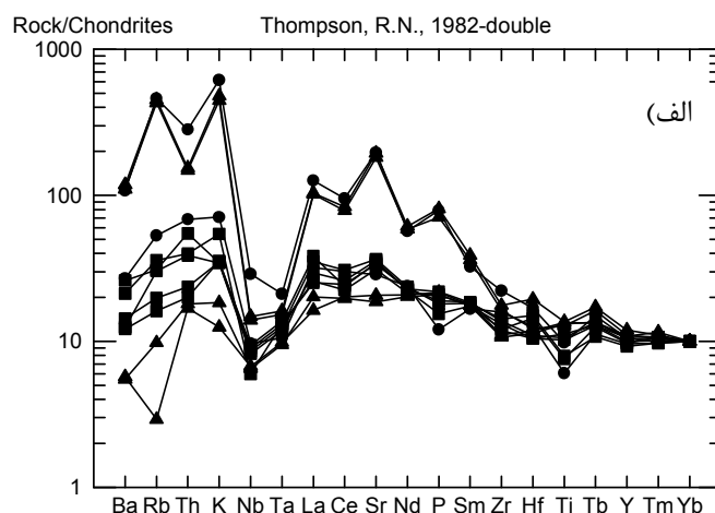
شکل ۷ الف- نمودار عنکبوتی جریان‌های گدازه‌ای منطقه‌ی راویز-زندیه، بهنجار شده براساس کندريت [۱۴]. نشانه‌ها مشابه شکل ۵.
