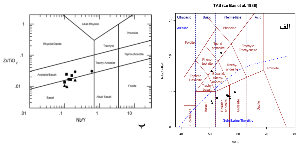
شکل ۵ الف) موقعیت سنگ‌های آتشفشانی منطقه‌ی راویز-زندیه در نمودار TAS [۷] و ب) موقعیت همین سنگ‌ها در نمودار \text{Zr}/\text{TiO}_2 - \text{Nb}/\text{Y} [۸]. نشانه‌ها: مثلث توپر: بازالت، دایره توپر: آندزیت و مربع توپر: بازالتیک آندزیت.
