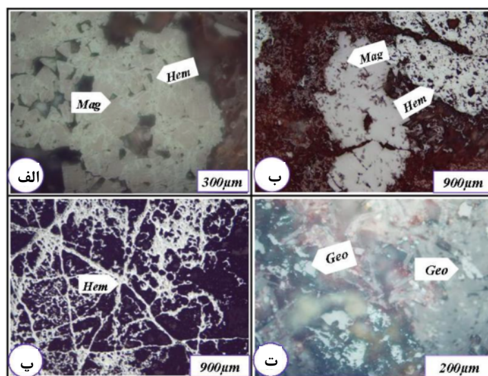
شکل ۸ الف) کانی مگنتیت که از مرکز در حال تبدیل شدن به هماتیت شعاعی است. ب) کانی مگنتیت در کنار قالبی از آن که به وسیله‌ی هماتیت جانشین شده است. پ) گوئیتیت‌های تشکیل شده طی فرایند دگرسانی از مگنتیت و هماتیت.
