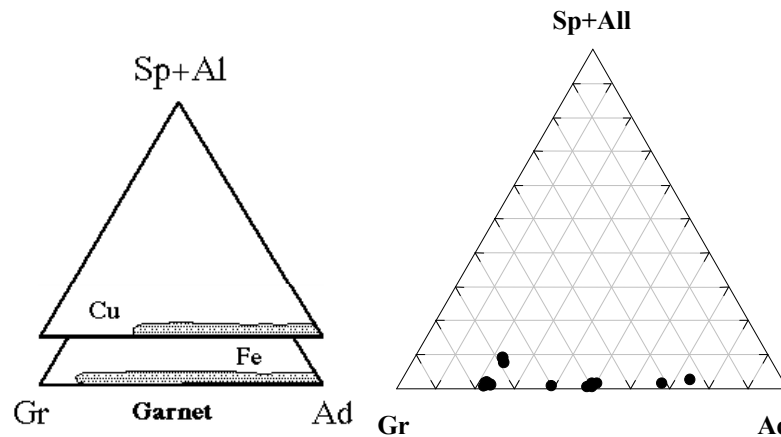
شکل ۹ نمودار توزیع ترکیب تجزیه‌های ریزکائنده‌ی الکترونی گارنت‌های اسکارن دره‌ی زرشک و مقایسه آن‌ها با ترکیب گارنت‌های انواع نهشته-های اسکارنی [۱۱،۱۰]. علائم اختصاری: Gr: گراسولار، Ad: آندرادیت، Sp: اسپسارتین، Al: آلماندن.
