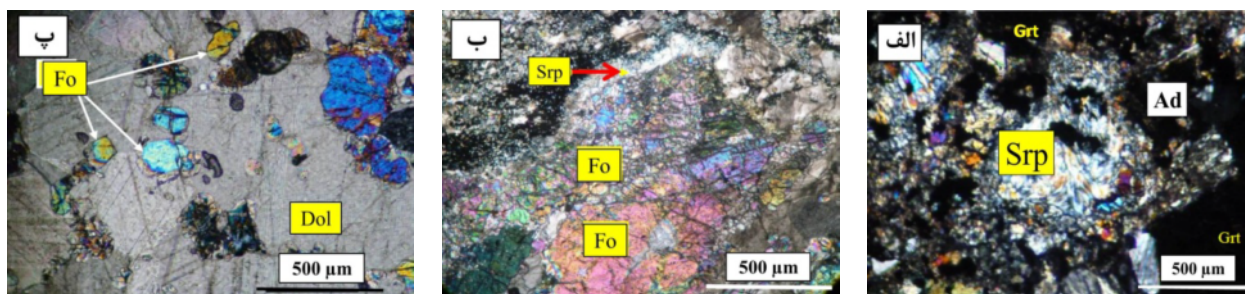
شکل ۷ الف جانشینی کامل اولیوین با سرپانتین و تشکیل شبرخت حاصل از آن ب: سرپانتینی شدن اولیوین و تشکیل بافت شبکه‌ای حاصل از آن در اسکارن منیزیمی. پ: درشت بلورهای اولیوین سالم با پیرامون گرد شده (Resorbed) در اسکارن منیزیمی.
