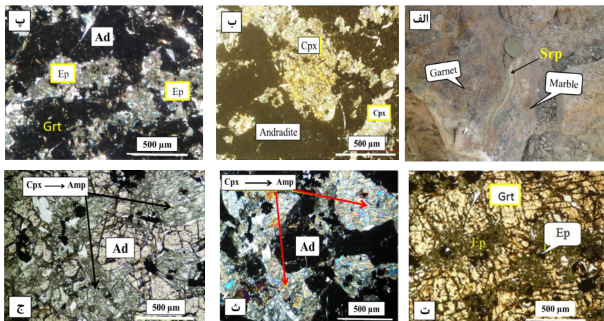
شکل ۵ الف: ساختار زونه متشکل از سرپانتین، مرمر و گارنت در زون گارنت-پروکسن اسکارن ب: جانشینی پروکسن با گارنت در زون گارنت - پروکسن. پ و ت: جانشینی گارنت با اپیدوت در زون گارنت-پروکسن (پ: نیکل عمود و ت: نیکل موازی). ث و ج: شبرخت پروکسن که کاملاً با آمفیبول رشته‌ای (اکتیلولیتی شدن) جایگزین شده است (ث: نیکل عمود و ج: نیکل موازی).
