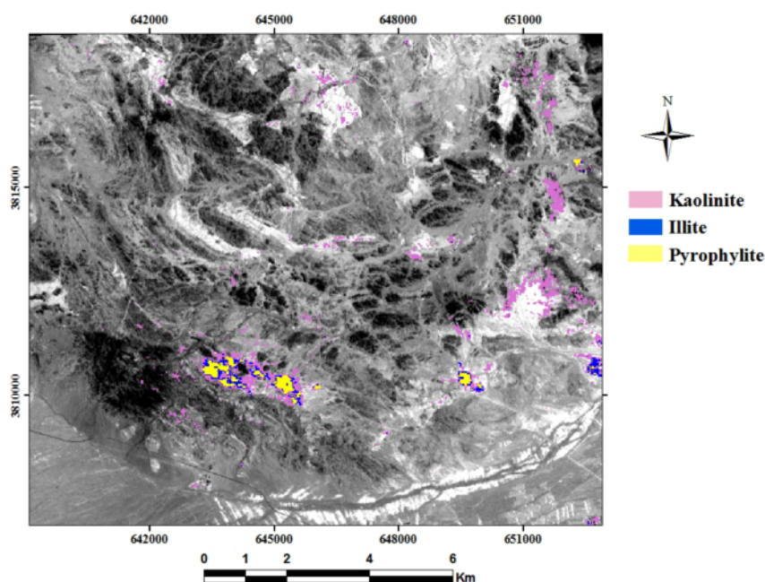
شکل ۲ کانی‌های رسی منطقه شمال غرب گناباد، که به روش نقشه‌برداری زاویه‌ی طیفی، منطبق بر زون‌های کائولینیتی موجود در منطقه پردازش شده است به خوبی نشان می‌دهد [۳].
