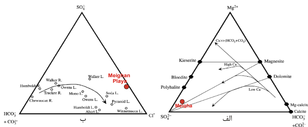
شکل ۷ نمودارهای مثلی اسپنسر [۳۹، ۴۰]. (الف) مسیرهای تکاملی شورابه و موقعیت پالای میقان روی نمودار \text{SO}_4^{2-} ، \text{HCO}_3^- ، \text{Mg}^{2+} . (ب) روند تکاملی شورابه‌ها، موقعیت انواع شورابه‌های مهم دنیا و پالای میقان بر روی نمودار سه تایی \text{SO}_4^{2-} ، \text{HCO}_3^- ، \text{Cl}^- .
