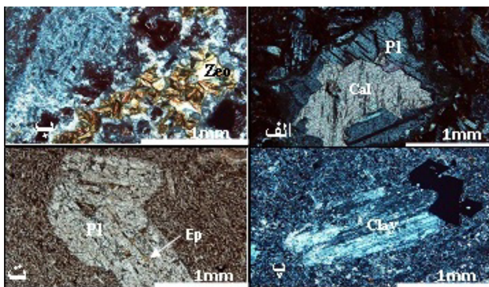
شکل ۷ الف) تبدیل پلاژیوکلاز به کلسیت در نور XPL ب) حفرات پر شده با ژئولیت در نور XPL پ) تبدیل پلاژیوکلاز به کانی رسی در نور PPL ت) تبدیل پلاژیوکلاز به اپیدوت در نور PPL، Ep: اپیدوت، Cal: کلسیت، Pl: پلاژیوکلاز، Zeo: ژئولیت، Clay: کانی رسی.
