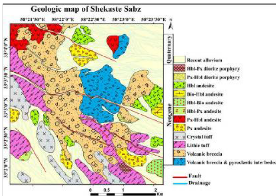
شکل ۵ نقشه‌ی زمین‌شناسی منطقه‌ی شکسته سبز.
