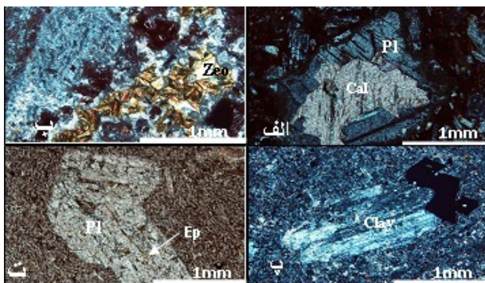
شکل ۷ الف) تبدیل پلاژیوکلاز به کلسیت در نور XPL ب) حفرات پر شده با ژئولیت در نور XPL پ) تبدیل پلاژیوکلاز به کانی رسی در نور PPL ت) تبدیل پلاژیوکلاز به اپیدوت در نور PPL، اپیدوت، Cal: کلسیت، Pl: پلاژیوکلاز، Zeo: ژئولیت، Clay: کانی رسی.
