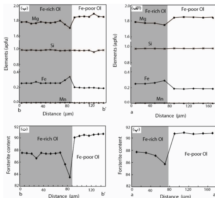
شکل ۳ (الف و ب): نمودار عناصر مختلف موجود در ترکیب کانی الیون نسبت به فاصله. موقعیت نقاط تجزیه شده در شکل ۲ و ت نشان داده شده است. (پ و ت): نمودار مقدار عضو انتهایی فورستریت در ترکیب کانی الیون نسبت به فاصله. موقعیت نقاط در شکل ۲ نشان داده شده است.
