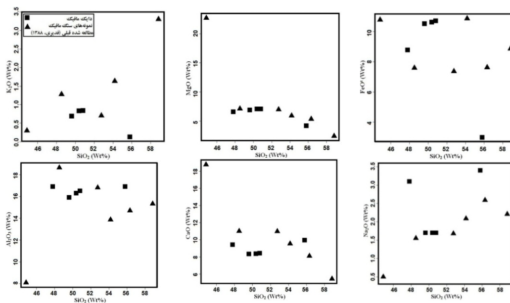
شکل ۶ نمودار اکسیدهای اصلی نسبت به سیلیس [۱۸]، برای نمونه‌های دایک مافیک و دیگر نمونه‌های مافیک موجود در منطقه.
