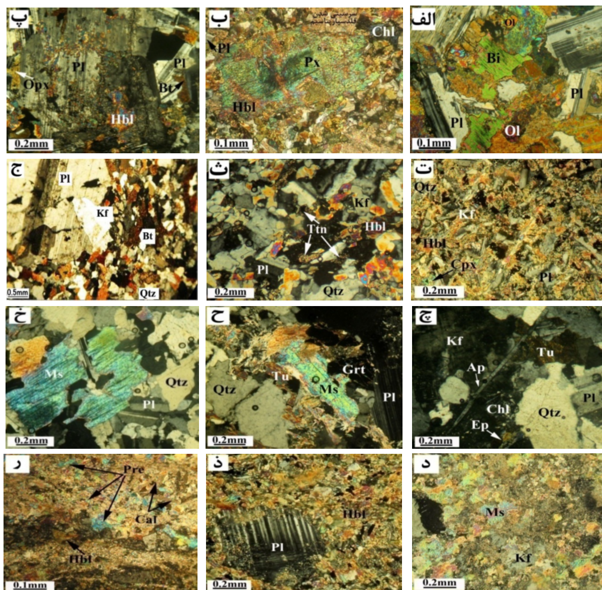
شکل ۳ تصاویر میکروسکوپی نمونه‌های برداشت شده از توده‌ی الوند: الف) الیون گابرو، ب) گابرو، پ) تشکیل کانی‌های ثانویه اورالیت در گابرو، ت) میکرودیوریت، ث) کوارتز دیوریت، ج) گرانیت پورفیری، چ) پگماتیت‌های تورمالین‌دار، ح) پگماتیت‌های تورمالین-موسکوویت-گرانیت‌دار، خ) پگماتیت‌های موسکوویت‌دار، د) آپلیت موسکوویت‌دار، ذ) مقطع میکروسکوپی یک دایک مافیک با ترکیب کوارتز دیوریت، ر) رگه پره‌نیت-کلسیت در یک کوارتز دیوریت، علائم اختصاری کانی‌ها بنابر [۱۹] انتخاب شدند.
