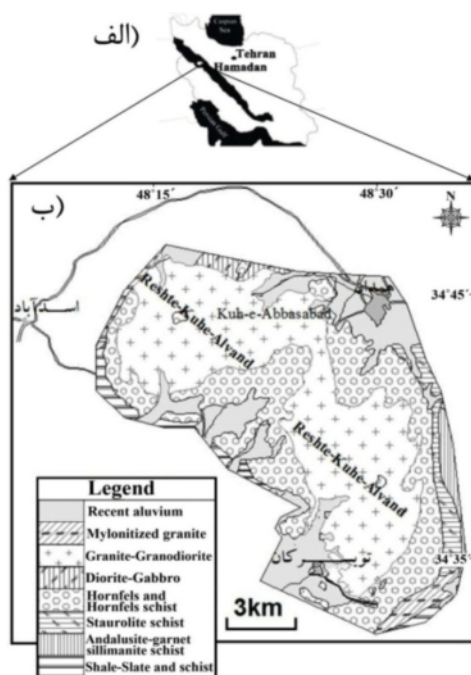
شکل ۱ الف) موقعیت منطقه‌ی مورد بررسی در زون سنندج سیرجان، ب) نقشه‌ی زمین‌شناسی ساده شده مجموعه‌ی پلوتونیک الوند (نقشه ۱:۲۵۰۰۰ چهار گوش همدان) با تغییرات از [۱۲].
