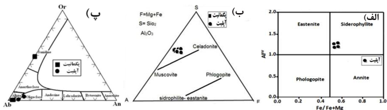
شکل ۱۳ الف) رده‌بندی بیوتیت‌ها بر اساس ترکیب شیمیایی آنها به روش [۲۶]، ب) رده‌بندی موسکوویت‌ها در پگماتیت‌ها و آپلیت‌های مورد بررسی بر اساس ترکیب شیمیایی، پ) رده‌بندی پلاژیوکلازها در پگماتیت‌ها و آپلیت‌های مورد بررسی بر اساس ترکیب شیمیایی [۲۶].
