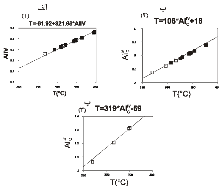
شکل ۷ الف- نقشه Al_{IV} نسبت به دما برگرفته از [۱] ب- نقشه Alc_{IV} نسبت به دما برگرفته از [۳۸] پ- نقشه Alc_{IV} نسبت به دما برگرفته از [۳۹]، توده پسته، ■، توده نقده = □.
