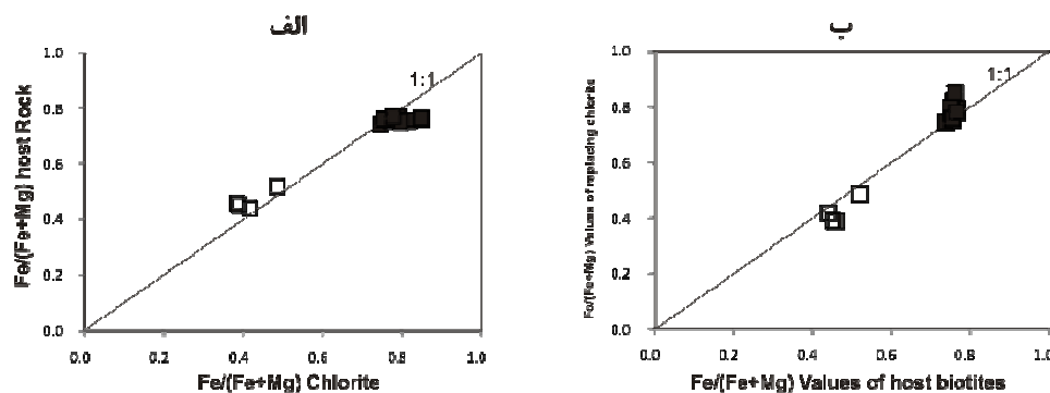
شکل ۴ الف) نقشه‌ی نسبت‌های Fe/(Fe+Mg) در نمونه‌های کلیت در مقابل نسبت‌های Fe/(Fe+Mg) در سنگ میزبان ب) پلات نسبت‌های Fe/(Fe+Mg) در کلیت‌های جانشین در برابر همین نسبت‌ها در بیوتیت میزبان در توده‌های نفوذی نقده و پسوه (توده‌ی پسوه=■، توده‌ی نقده=□).
