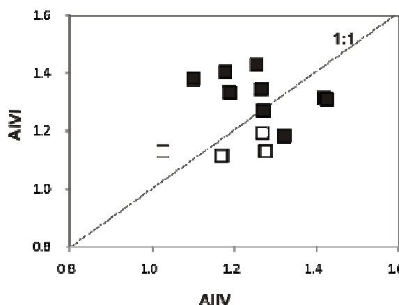
شکل ۶ نقشه ی مقدار Al چاروجهی نسبت به Al هشت وجهی در کلریت های سنگ های گرانیتی توده های پسوه و نقده، توده پسوه، توده نقده. □ = توده نقده، ■ = پسوه.
