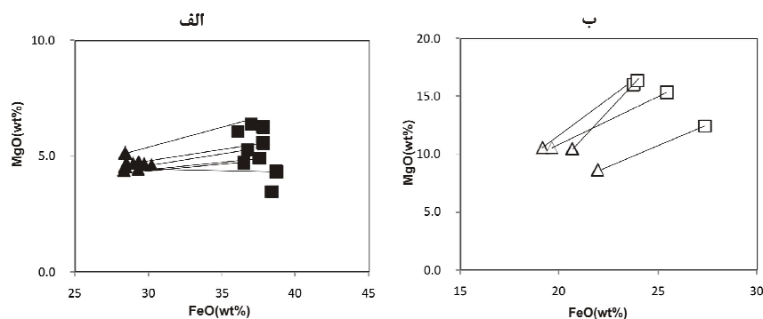
شکل ۵ نقشه‌ی مقادیر FeO نسبت به MgO در نمونه‌های کلیت و نمونه‌های بیوتیت میزبان در سنگ‌های گرانیتوئیدی توده‌های پسوه و نقده (الف- توده‌ی پسوه، کلیت=■، بیوتیت=▲) (ب- توده‌ی نقده □ = کلیت، ▲ = بیوتیت).
