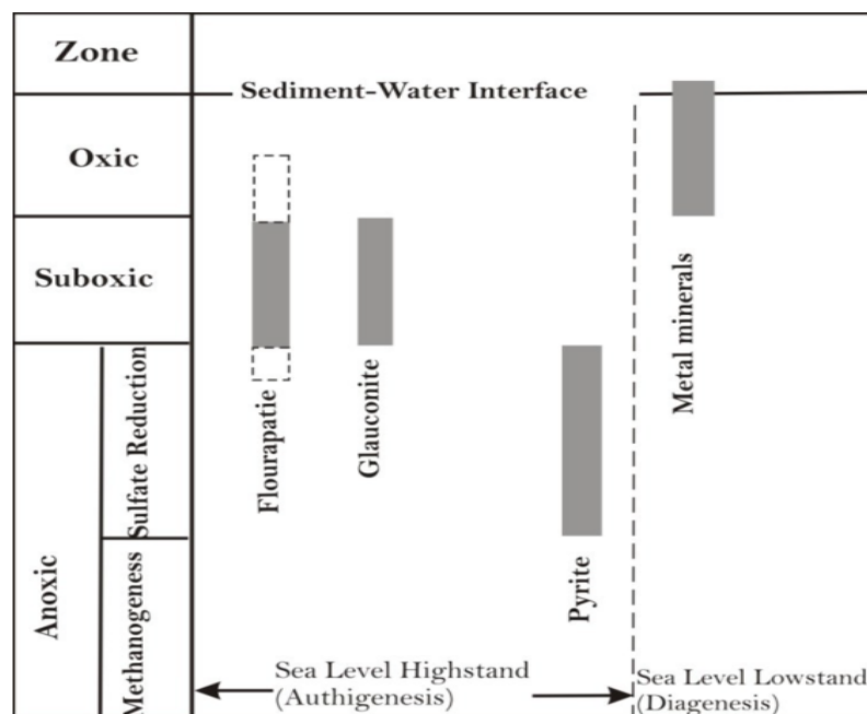
شکل ۶ توالی پاراژنزی برای کانای‌های مشاهده شده در دو کانسار کوه سفید و بناری [۱۶].
