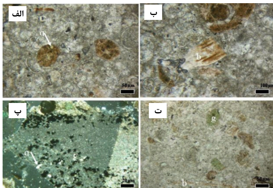
شکل ۸ پلت فسفاتی نیمه‌زاویه‌دار (الف)، قطعه استخوان ماهی بی‌شکل از سازند پابده در کانسار بناری (ب)، اینتراکلاست که دانه کوارتز (رنگ روشن) و پیریت (سیاه رنگ) در آن پراکنده است (پ)، گلوکونیت با گرد شدگی که در آن آثار شکستگی دیده می‌شود (ت). (علائم اختصاری: کوارتز (q)، قطعه استخوان (b)، گلوکونیت (g)). (مقاطع الف، ب و د، در PPL و مقطع ج در XPL).
