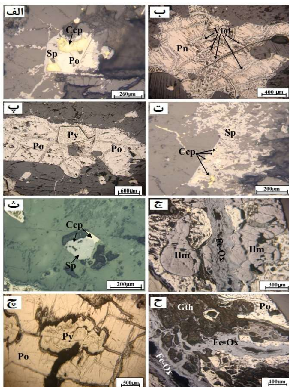
شکل ۵ تصاویر میکروسکوپی از کانه‌های سولفیدی در نمونه‌های مورد بررسی (ppl). الف) ادخال کالکوپیریت در پیروتیت و اسفالریت که از حاشیه جانشین پیروتیت شده است. ب) پنتلاندیت که در اثر دگرسانی برونزادی به ویولاریت تبدیل شده است، پ) پیریت نسل اول نیمه شکل‌دار، که به صورت ادخال در پیروتیت مشاهده می‌شود، ت و ث) کانه اسفالریت که دارای بیماری کالکوپیریت است، ج) کانه اکسیدی ایلمنیت به رنگ خاکستری تیره و هیدروکسی / اکسیدهای آهن حاصل از اکسایش پیروتیت، چ) دگرسانی برونزادی پیروتیت به پیریت که منجر به تشکیل بافتی ثانویه به نام چشم پرنده شده است، ح) هیدروکسی / اکسیدهای آهن و گوتیت حاصل از اکسایش پیروتیت که به صورت حاشیه‌هایی در اطراف پیروتیت و رگه‌هایی که بلورهای پیروتیت را قطع کرده‌اند مشاهده می‌شوند. (پیروتیت: Po، پنتلاندیت: Pn، کالکوپیریت: Ccp، پیریت: Py، ترویلیت: Tro، اسفالریت: Sp، ایلمنیت: Ilm، مگنتیت: Mag، ویولاریت: Viol، گوتیت: Gth)
