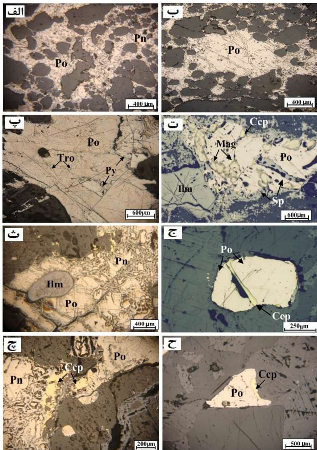
شکل ۴ تصاویر میکروسکوپی از کانه‌های سولفیدی در نمونه‌های مورد بررسی (ppl). الف) کانه‌های سولفیدی پیروتیت و پنتلاندیت که کانی‌های سیلیکاتی را در برگرفته، ب) پیروتیت که در بیشتر نمونه‌های منطقه حضور دارد، پ) تیغه‌های به رنگ روشن ترویلیت و ادخال پیریت در پیروتیت، ت) پیروتیت دارای ادخال‌هایی از کالکوپیریت، اسفالریت و مگنتیت، ث) پیروتیت و پنتلاندیت که جانشین ایلمنیت شده‌اند، ج) هم رشدی پیروتیت و کالکوپیریت، چ) کالکوپیریت به صورت بی شکل که فضای بین بلورهای پیروتیت را پر کرده است، ح) کالکوپیریت که از حاشیه جانشین پیروتیت شده است.
