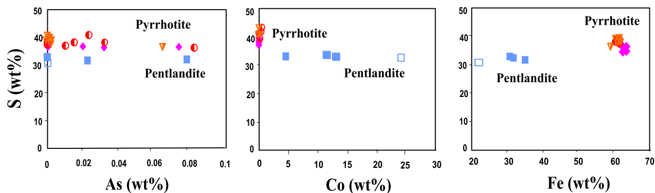
شکل ۸ نقشه‌ی تمرکز عناصر \text{Fe} , \text{Co} , \text{As} و \text{S} نسبت به گوگرد برای پیرویت و پنتلاندیت نمونه‌های مافیک میشو [۱۵].
