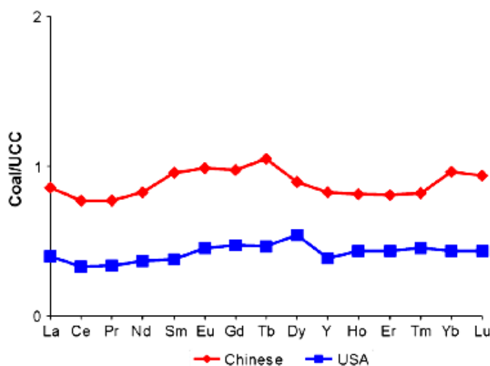
شکل ۳ نمودار میانگین عناصر خاکی نادر در زغال‌های چین و آمریکا ۱ [۳].
