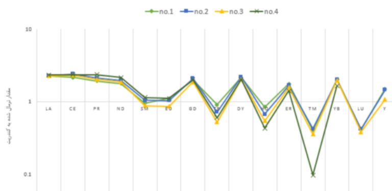
شکل ۵ الگوی توزیع عناصر خاکی نادر در نمونه‌های شماره ۱ تا ۴ معدن کارمزد.
