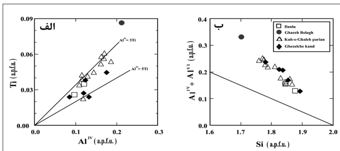
شکل ۴ الف) ترکیب شیمیایی کلینوپروکسن‌های منطقه‌ی شمال شرق قروه روی نمودار تغییرات Al^{IV} -Ti، ب) ترکیب شیمیایی کلینوپروکسن‌های منطقه‌ی شمال شرق قروه روی نمودار Al-Si.
