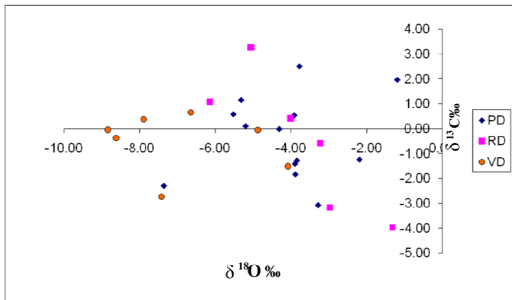
شکل ۸. نمودار \delta^{13}\text{C} نسبت به \delta^{18}\text{O} در انواع دولومیت‌های سازند پادها. دولومیت‌های نوع PD و RD دارای گستره‌ی تقریباً مشابهی است ولی دولومیت‌های نوع VD از گستره‌ای مجزا و از مقادیر منفی‌تری برخوردار است.
