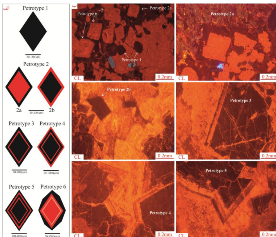
شکل ۴ انواع سنگ‌گونه‌های شناسایی شده در دولومیت‌های نوع VD. (الف) شکل نموداری از انواع سنگ‌گونه‌ها. (ب) تصاویر کاتدولومینسانس از انواع سنگ‌های شناسایی شده در دولومیت‌های نوع VD. توضیحات هر کدام از انواع سنگ‌ها در متن آورده شده است.
