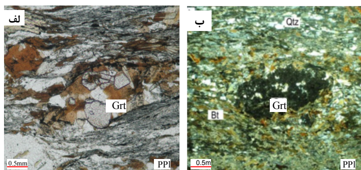
شکل ۲ مقطع میکروسکوپی گارنت شیبست‌های منطقه‌ی بلند پرچین. (الف) گارنت‌های خود شکل بدون شواهد مبنی بر دگرگونی برگشتی و فاقد منطقه بندی شیمیائی (ب) بلورهای اتول گارنت دارای ادخال‌های فراوان و حواشی بریده.
