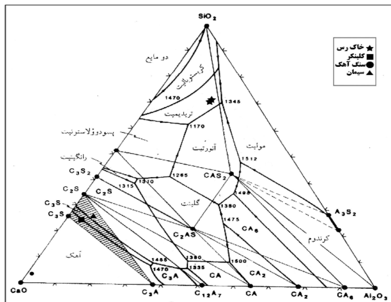
شکل ۱۹ روابط فازی در فشار یک اتمسفر در سیستم کربن دیوکسید کربن بدون آب C - A - S ، نشان دهنده‌ی موقعیت ترسیمی سنگ آهک، خاک رس، کلینکر و سیمان پرتلند کارخانه‌ی سیمان نکاء.
