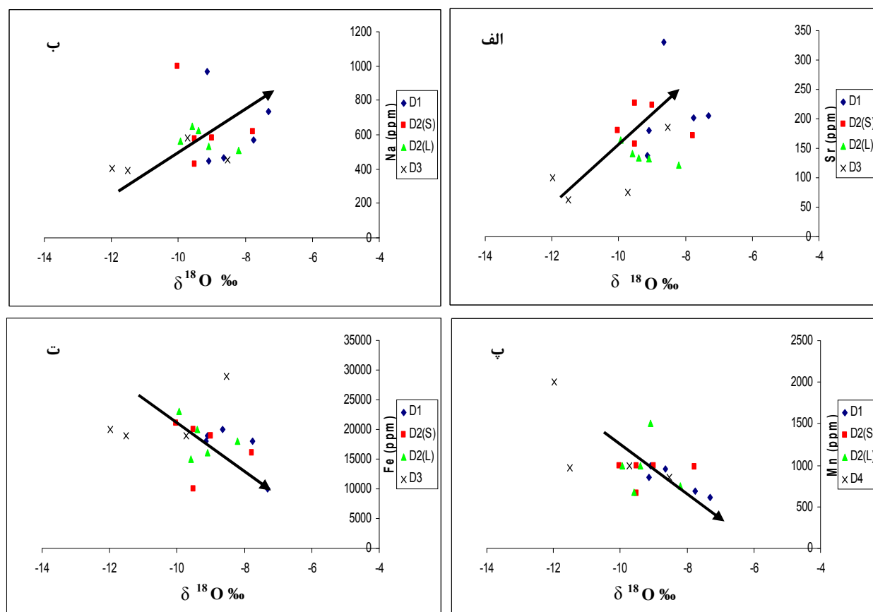
شکل ۷ روند تغییرات عناصر Na، Sr، Fe و Mn در مقابل \delta^{18}\text{O} در انواع مختلف دولومیت‌های سازند درنجال.
