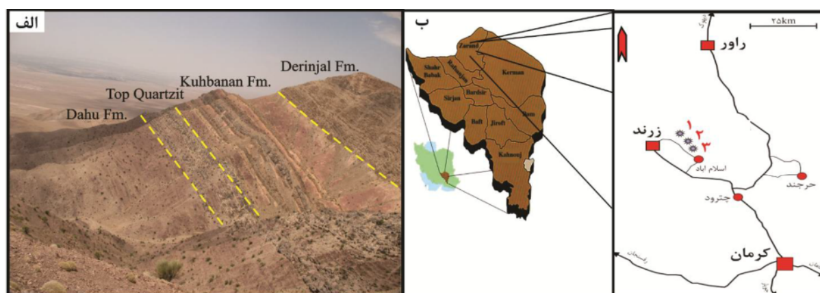
شکل ۱ الف) تصویر صحرایی از دنباله‌ی نهشته‌های کامبرین در شمال غرب کرمان (دید به سمت غرب). ب) موقعیت جغرافیایی برش‌های مورد بررسی در گستره‌ی زرنند. ۱: گزوه‌ی (۳۱° ۳۰' عرض شمالی و ۴۱° ۵۶' طول شرقی)؛ ۲: گتکوه‌ی (۴۸° ۳۰' عرض شمالی و ۴۲° ۵۶' طول شرقی)؛ ۳: داهوئیه (۴۸° ۳۰' عرض شمالی و ۴۲° ۵۶' طول شرقی).
