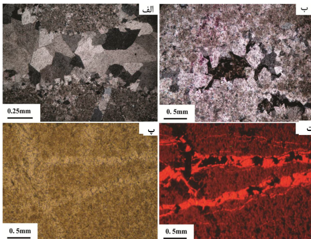
شکل ۵ تصاویر میکروسکوپی دولومیت نوع ۳. الف) دولومیت‌های درشت بلور و یکنواخت D_3 پر کننده رگه‌های انحلالی. از دیواره به سمت مرکز بلورها از حالت خودشکل به نیمه شکل‌دار و بی شکل تغییر می‌کند (XPL). ب) بلورهای درشت D_3 شکل‌دار تا نیمه شکل‌دار پر کننده حفرات (XPL). پ) دولومیت‌های درشت بلور نیمه شکل‌دار پر کننده رگه (PPL). ت) تصویر C در CL. لومینسانس‌های درخشانده و مات، نشان دهنده تغییر شرایط شیمیایی در زمان تبلور دولومیت است.
