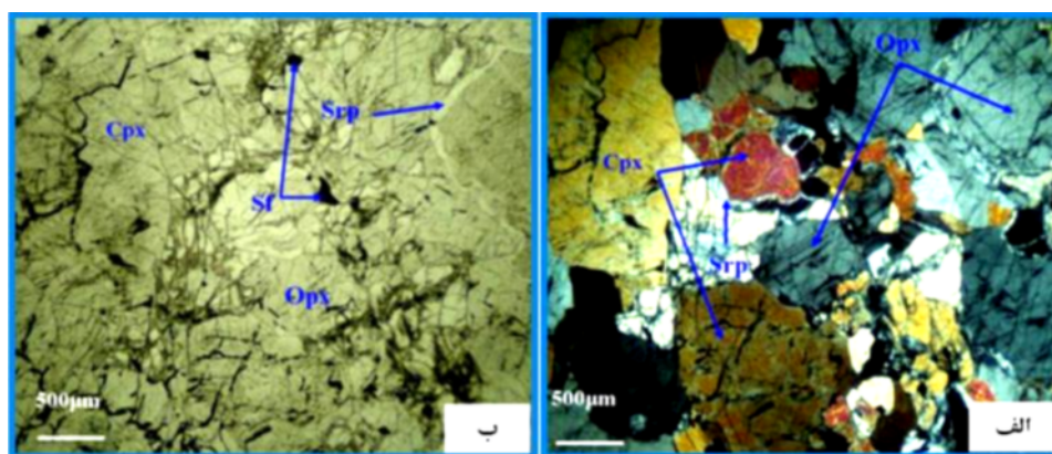
شکل ۷ کانی‌های سولفیدی (Sf)، ارتوپیروکسن (Opx) و کلینوپیروکسن (Cpx) در سنگ‌های فاریاب (سرپانتین = Srp) (الف نور XPL و ب نور PPL).
