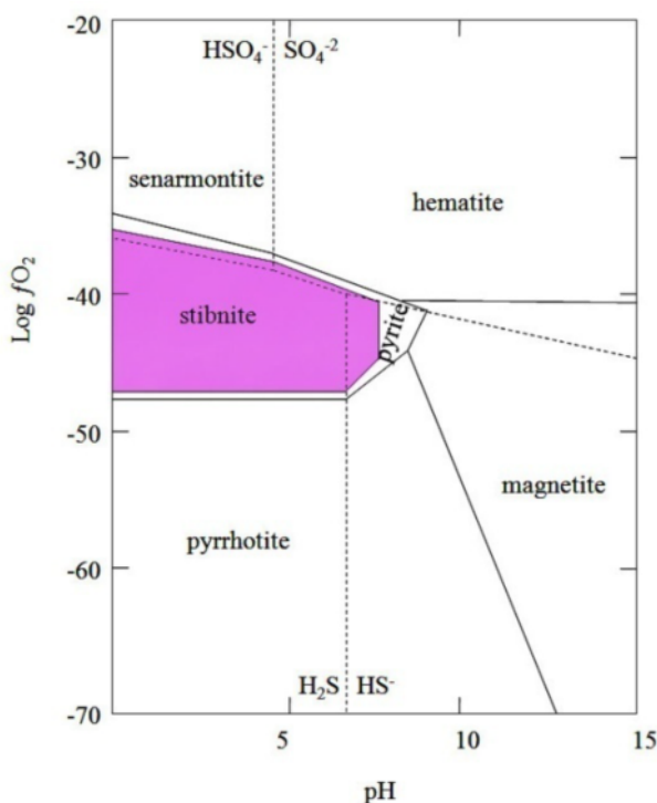
شکل ۱۴ نمودار pH- logfO2 ترسیم شده در ۲۰۰ درجه‌ی سانتیگراد و \Sigma a_s = ۰/۰۱ که نشان دهنده‌ی گستره‌ی پایداری استیبنیت در سیستم Fe-Sb-S-O در کانسار شورچاه است.
