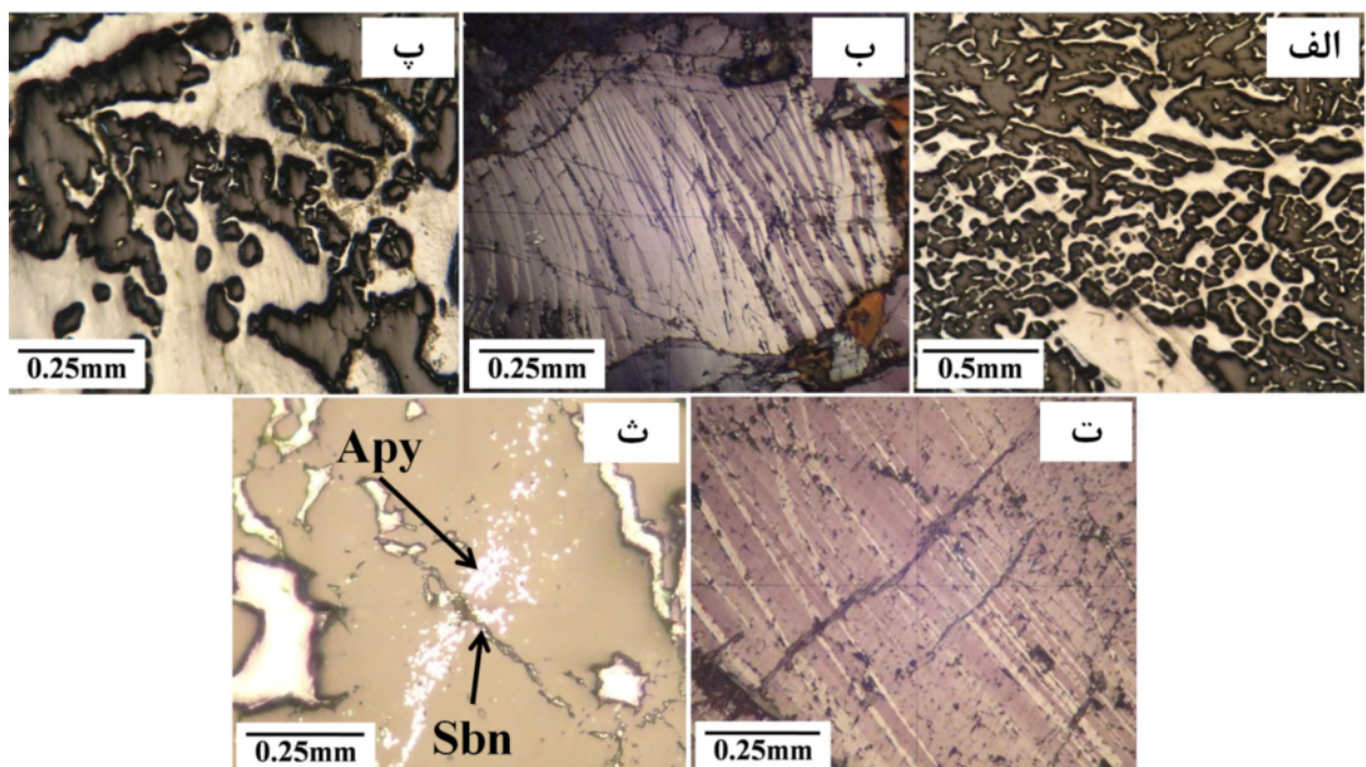
شکل ۹ مقاطع میکروسکوپی الف: استیبنیت‌های اسکلتی (PPL)، ب: ماکل پلی‌سنتیک در استیبنیت‌ها (XPL)، پ: بافت پرکننده‌ی فضای خالی استیبنیت‌ها (PPL)، ت: استیبنیت‌های توده‌ای (XPL)، ث: رگه‌ای از آرسنوپیریت که با رگه‌ای از استیبنیت قطع شده است (PPL). Apy: آرسنوپیریت، Sbn: استیبنیت.
