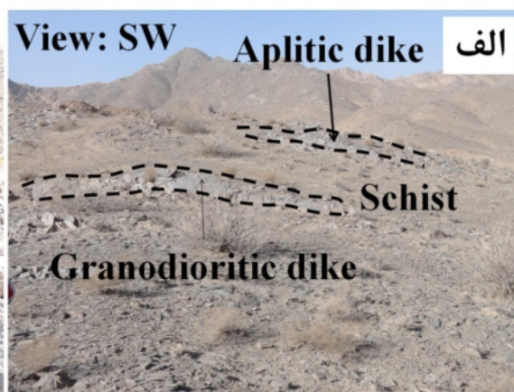
شکل ۲ الف: نمایی از دایک‌های آپلیتی و گرانودیوریتی در میان شیست‌های کانسار شورچاه، ب: نمایی از نوارهای گرانودیوریتی نفوذ کرده در میان شیست‌های بخش شورچاه.
