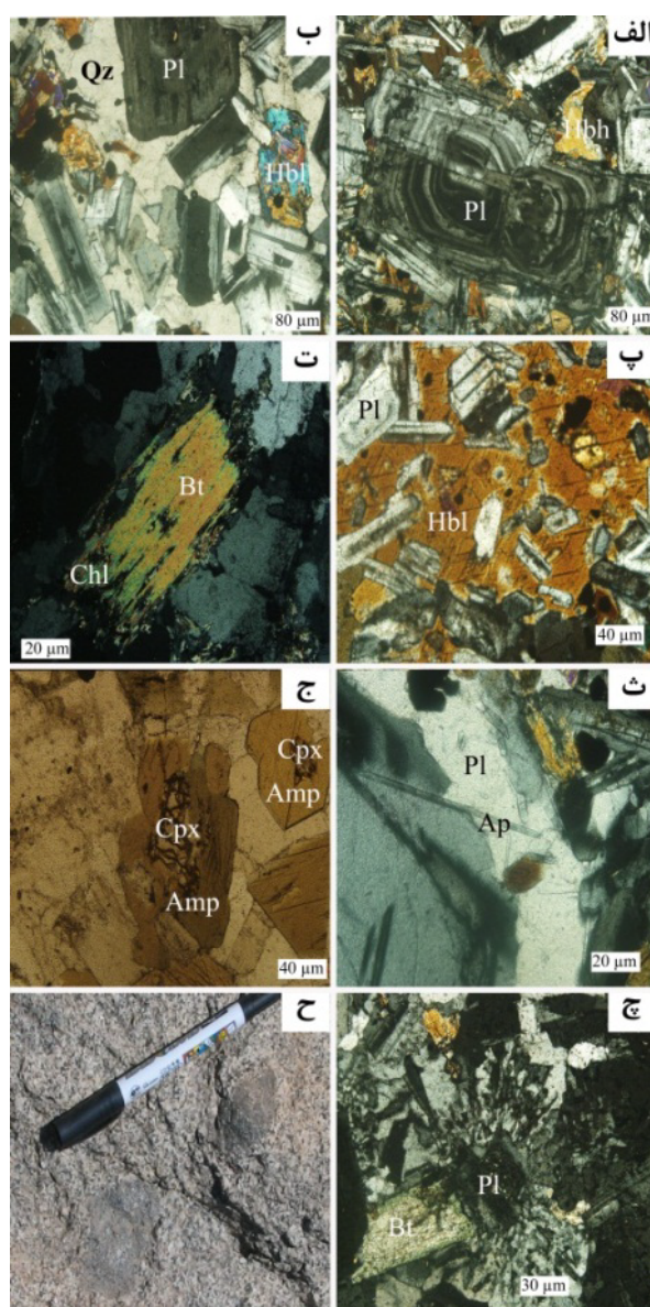
شکل ۲ الف) منطقه‌بندی در پلاژیوکلاز در سنگ گابرو دیوریت (XPL، ب) ادخال‌هایی از دانه‌های کوچک آمفیبول و پلاژیوکلاز در بلور کوارتز در کوارتز دیوریت (XPL، پ) آمفیبول با ادخال‌هایی از کانی کدر و پلاژیوکلاز در گابرو دیوریت (XPL، ت) بیوتیت تجزیه شده به کلریت در تونالیت (XPL، ث) آپاتیت سوزنی در گابرو دیوریت (XPL، ج) آمفیبول جایگزین شده به جای پیروکسن در دیوریت (XPL، چ) بافت ریزدانه-ای در کوارتز مونزونیت (XPL، ح) شکل‌های بیضوی و گرد شده برونوم ریز دانه‌ای منطقه شرق نابر.
