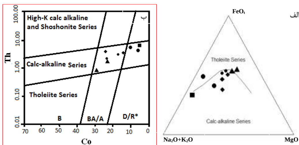
شکل ۶ الف) موقعیت نمونه‌های مورد بررسی بر الف) نمودار AFM [۵] و ب) نمودار \text{Co} نسبت به \text{Th} [۶] که همه نمونه‌ها به جز دو نمونه که به احتمال بسیار دگرسان شده‌اند در گستره سری آهکی قلیایی قرار دارند.
