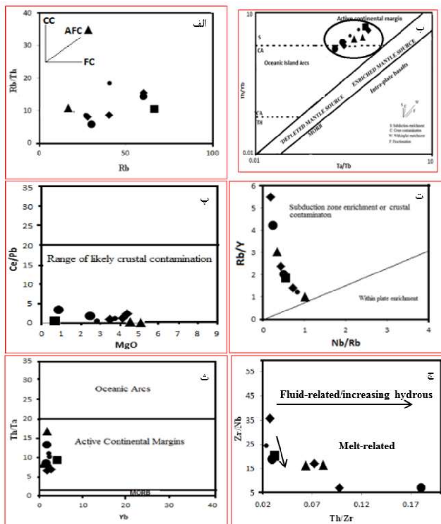
شکل ۱۰ نمودارهای تغییرات نسبت‌های عناصر برای تشخیص خاستگاه: الف) نمودار Rb نسبت به Rb/Th (ب) نمودار Ta/Yb نسبت به Th/Yb، پ) نمودار MgO نسبت به Ce/Pb [۲۶]، ت) نمودار Nb/Rb نسبت به Rb/Yb (ث) نمودار Yb نسبت به Th/Ta، ج) نمودار Th/Zr نسبت به Zr/Nb [۲۷]. (S) فرورانش، CA: آهکی قلیایی، TH: تولیتی، CC: آلودگی پوسته‌ای، AFC: هضم، جدایش و تبلور، FC: جدایش بلورین.
