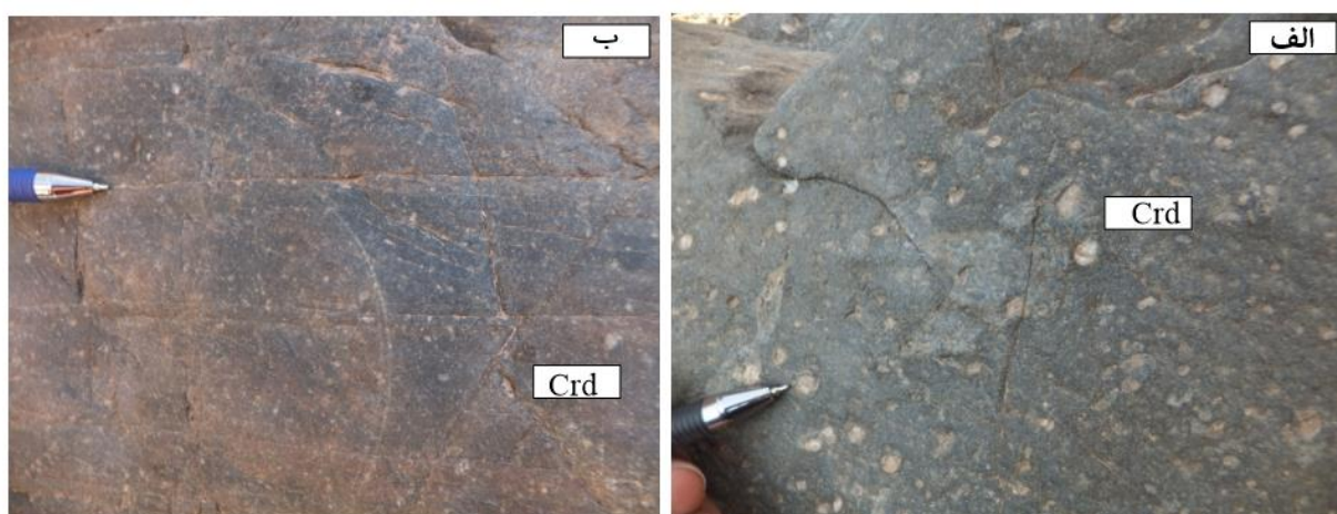
شکل ۴ نمونه‌های دستی از اسلیت لکه‌دار در هاله دگرگونی میشو. کانی‌های کردیریت به شکل لکه‌های سفید رنگ در سنگ دیده می‌شوند.
