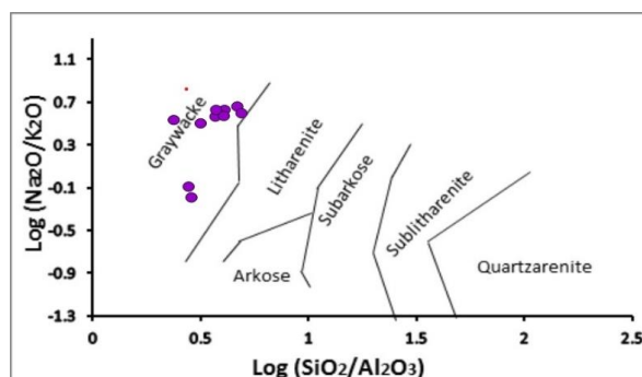
شکل ۱۴ ترکیب سنگ مادر هورنفلس‌ها در هاله دگرگونی مجاورتی میشو بر پایه نمودار Log (Na2O/K2O) نسبت به Log (SiO2/Al2O3) [۹]. مرزها توسط داده‌های مرجع [۱۰] اصلاح شده است. ترکیب سنگ مادر در سنگ‌های دگرگونی مجاورتی میشو در گستره ماسه سنگ تیره است.
