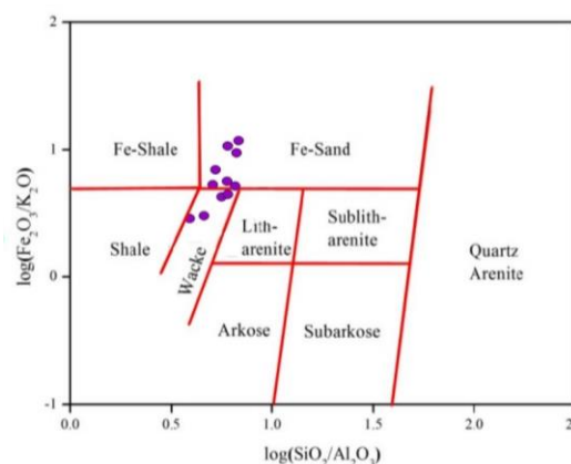
شکل ۱۵ ترکیب سنگ مادر انواع سنگ‌های هورنفلسی در هاله دگرگونی مجاورتی میشو براساس نمودار Log (Fe2O3/K2O) نسبت به Log (SiO2/Al2O3) [۱۰] که نمونه‌های مورد بررسی در گستره ماسه سنگ آهن‌دار تا ماسه سنگ تیره قرار دارند.
