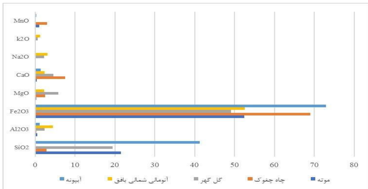
شکل ۱۴ نمودار چند عنصری برای مقایسه درصد اکسیدهای اصلی در کانسنگ آبونه با برخی از معادن آهن در پهنه سنج - سیرجان و ایران مرکزی.
