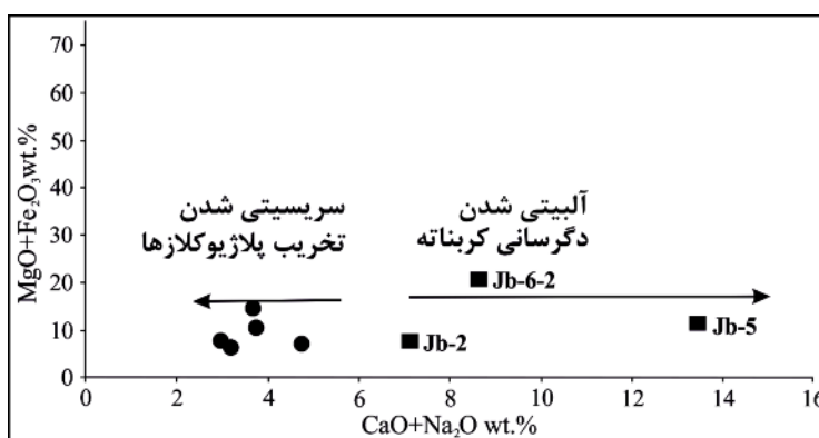
شکل ۵ تفکیک رخساره‌های دگرسان بر حسب \text{CaO} + \text{Na}_2\text{O} در برابر \text{MgO} + \text{Fe}_2\text{O}_3 در نمونه‌های مورد بررسی، (نمودار پایه از [۱۳]).
