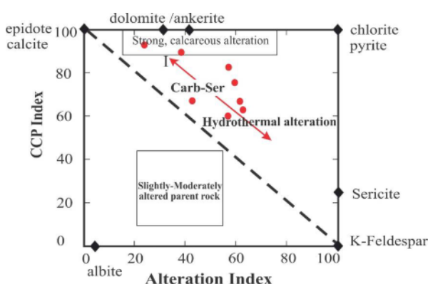
شکل ۷ نمودار جعبه‌ای دگرسانی [شاخص دگرسانی ایشیکاوا ( AI ) نسبت به شاخص دگرسانی کلریت-کربنات-پیریت ( CCPI )] برای داده‌های تجزیه‌ی شیمیایی منطقه‌ی مورد بررسی. روند اصلی دگرسانی با روند I (دگرسانی سیرسیتی-کربناته) نشان داده شده است.
