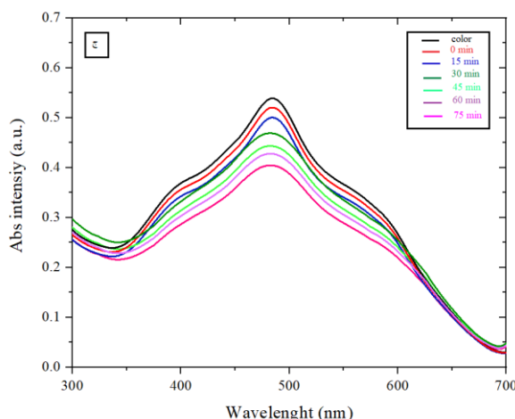
شکل ۸. بازده تخریب رنگ متیل قرمز برای فوتوکاتالیزور \text{Ag}_2\text{S}/\text{ZnS}/\text{Fe}_3\text{O}_4 زیر تابش نور فرابنفش در مدت ۷۵ دقیقه در (الف) \text{pH}=3 ، (ب) \text{pH}=7 و (ج) \text{pH}=9 .
