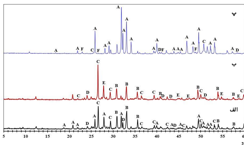
شکل ۲ الگوی پراش پرتوی ایکس الف (خوراک، ب) باطله و پ) ماده عیار ( \text{Ca}_5(\text{PO}_4)_3\text{F} ، (A: آپاتیت)، ( \text{Fe}_2\text{O}_3 ، B: هماتیت)، ( \text{SiO}_2 ، C: کوارتز)، D: \text{CaMg}(\text{CO}_3)_2 ، دولومیت)، ( \text{NaAlSi}_3\text{O}_8 ، E: آلبیت)، \text{CaCO}_3 (کلسیت)، F: کلسیت).
