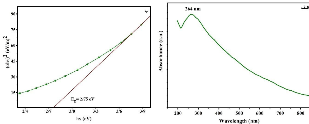
شکل ۷ الف) طیف جذبی نانوذرات \text{La}_2(\text{WO}_4)_3 ، ب) نمودار (\alpha h\nu)^2 نسبت به h\nu .
