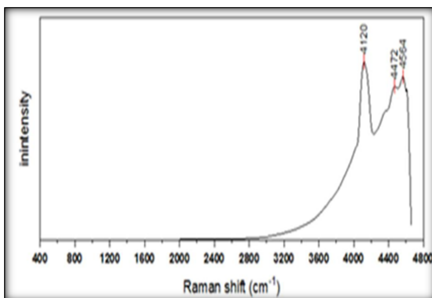
شکل ۱۵ طیف رامان زمرد دره پنچشیر افغانستان.
