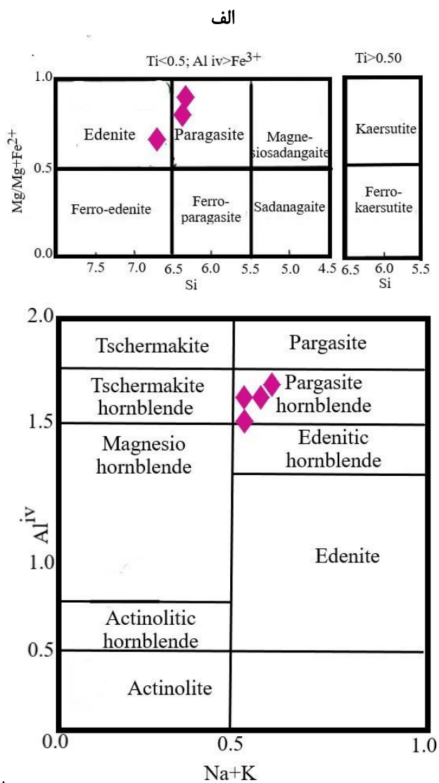
شکل ۷ رده‌بندی آمفیبول‌های موجود در سنگ‌های منطقه براساس الف) در نمودار مرجع [۴۳] و ب- نمودار پیشنهادی مراجع [۴۴، ۴۳]
