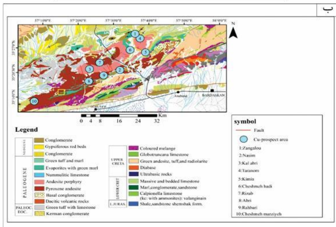
شکل ۱ الف) موقعیت منطقه شمال غرب بردسکن در پهنه ایران مرکزی [۷، ۸]؛ ب) موقعیت قابلیت‌های معدنی مس شمال غرب بردسکن بر نقشه ۱:۲۵۰۰۰ کاشمر برگرفته از مرجع [۹] همراه با تغییرات.
