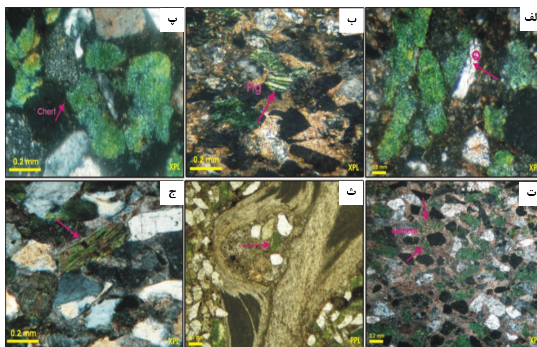
شکل ۷ انواع جانیشینی گلاکونی. الف: در کوارتزهای ماسه‌سنگ‌های برش باغک، ب: در پلاژیوکلازهای ماسه‌سنگ‌های برش شوربجه، پ: در خرده-سنگ‌های چرتی ماسه‌سنگ‌های برش باغک، ت: در سیمان کربناتی ماسه‌سنگ‌های برش شوربجه، ث: در پوسته‌ی اسکلتی ماسه‌سنگ‌های فسیل‌دار برش باغک، ج: در کانی‌های ورقه‌ای ماسه‌سنگ‌های برش شوربجه.
