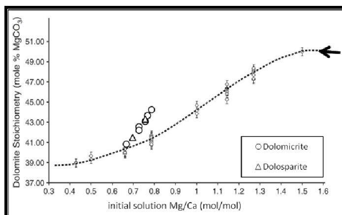
شکل ۶ روند تغییرات عنصرسنجی دولومیت‌های تشکیل شده از آهک‌های اولیه در شرایط آزمایشگاهی در ارتباط با نسبت مولی Mg^{2+}/Ca^{2+} سیال اولیه (علامت پیکان)، با توجه به ارتباط بین عنصرسنجی و نسبت Mg^{++}/Ca^{++} شاره‌ی اولیه، نشان می‌دهند که دولومیت‌های سازند شهبازان از شاره‌هایی با نسبت Mg^{2+}/Ca^{2+} پایین (در حدود ۱) شکل گرفته باشند.
