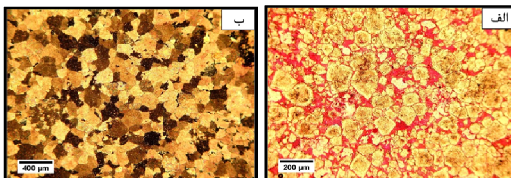
شکل ۶ الف) دولومیت‌های بلوری متوسط در سازند شهبازان با بافت مسطح نیمه شکل‌دار با خاموشی مستقیم که در زمینه‌ای از کلسیت اسپاری شناورند. (نمونه رنگ‌آمیزی شده، PPL، برش قورچ‌باشی، KKQ-36)، ب) دولومیت‌های متوسط تا درشت بلور با خاموشی موجی سازند شهبازان با بافت غیرمسطح بی‌شکل تا نیمه شکل‌دار. (نمونه رنگ‌آمیزی شده، XPL، برش قورچ‌باشی، KKQ-21).
